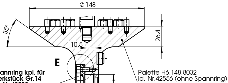
Spannvorrichtung für Werkstück Gr. 14
