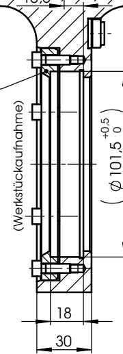
Spannring kpl. für Werkstück Gr. 18 Id.-Nr.42554
