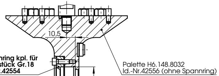
Spannvorrichtung für Werkstück Gr. 18
