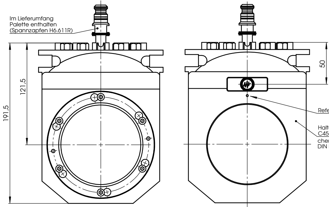
Spannvorrichtung für Werkstück Gr. 14
