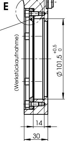
Spannring kpl. für Werkstück Gr. 14 Id.-Nr.42552
